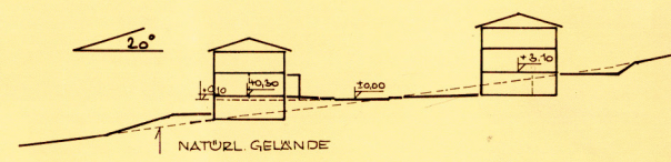
SCHNITT A-B 1:500
